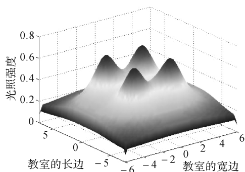
图 1-3 反射情况下教室光照强度示意图
