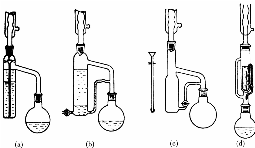
图 1.1 连续萃取装置
