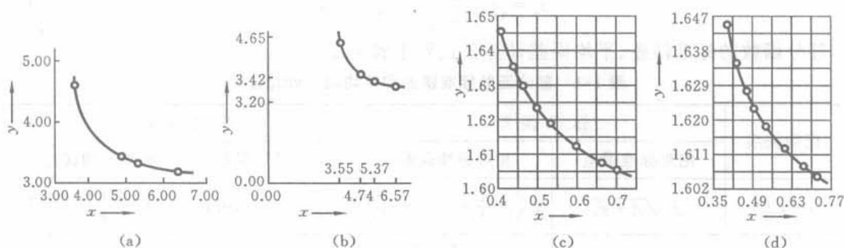
图 1-3 作图法表示实验数据
