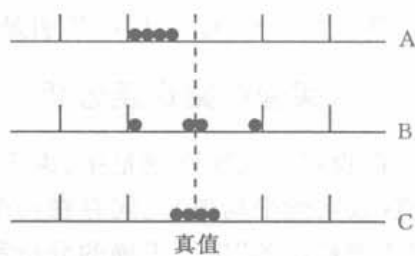
图 1-2 精密度和准确度
