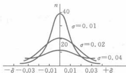
图 1-1 偶然误差正态分布曲线
