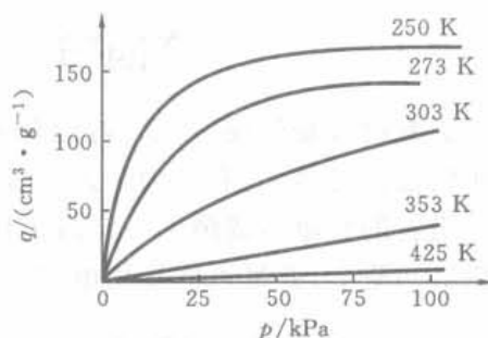
图 1-4 曲线的绘制方法
