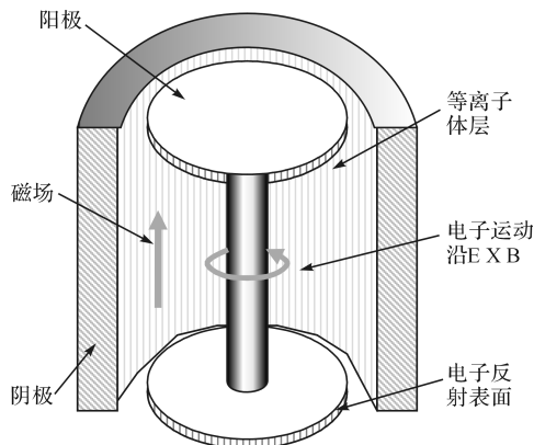
图 1-6 磁控溅射
