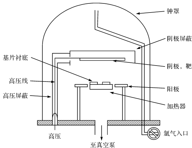
图 1-5 简单的溅射装置
