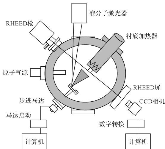
图 1-7 激光熔蒸分子束外延装置
