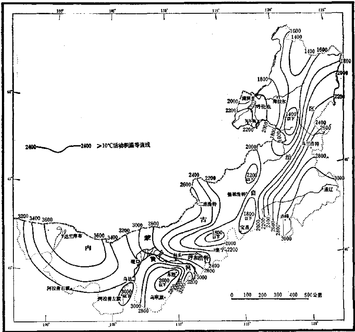
图3 \geq 10^{\circ}\text{C} 全年活动积温分布图
