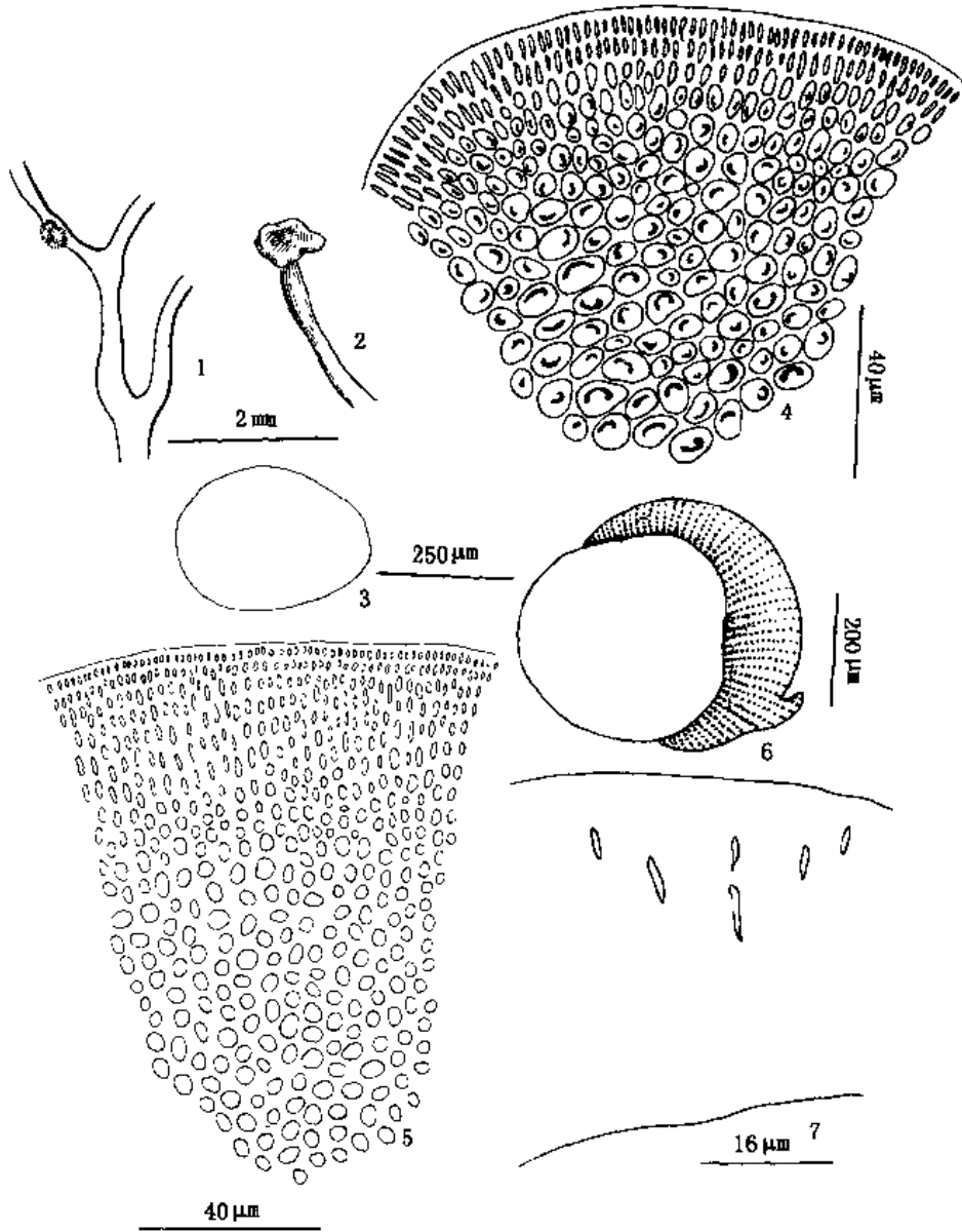
图 1 帚状伊谷藻 Ahnfeltia fastigiata (Post et Ruprecht) Makienko (AST 60-1447) 1. 2. 果孢子体外形图; 3. 中轴横切面观; 4. 5. 部分中轴横切面观; 6. 果孢子体横切面观; 7. 雌性孢子堆中的果胞。
