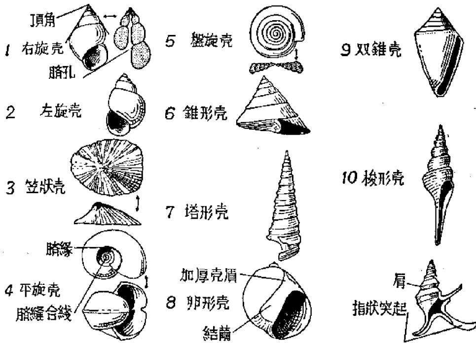
图5 几种螺壳的形状(从 Moore)
