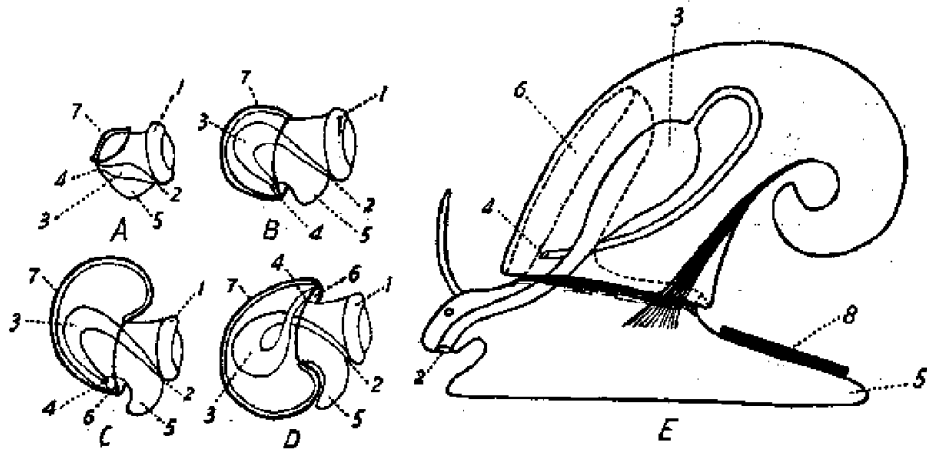
图3 腹足类个体发育期间内脏囊发生扭转的顺序及其成年体的图解 A. 未经扭转的幼虫； B. 消化管发生扭转而螺壳仍为罩状； C. 内脏囊逐渐扭转； D. 内脏囊扭转180°，肛门及外套腔移向前端的背侧； E. 成年腹足动物构造图解(左视) 1. 游泳器官，2. 口，3. 消化管，4. 肛门，5. 足，6. 外套腔，7. 胚胎期之壳，8. 口盖 (从 Давишвили)
