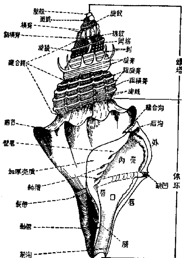
图 6 腹足类螺壳各部构造及纹饰综合图 (从 Shrock and Twenhofel)
