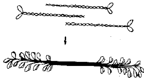
图 8 肌球蛋白分子及其聚合成的粗丝
