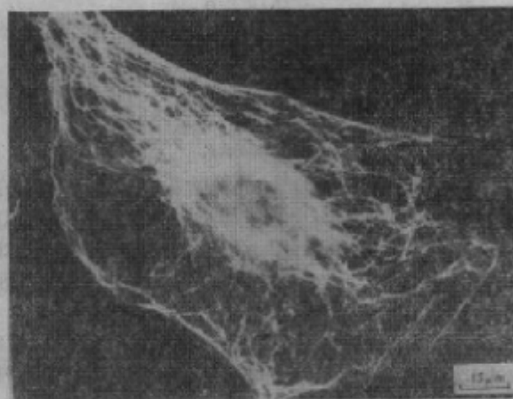
图4 用荧光免疫技术见到的细胞中微管的分布 微管好似由核区放射出的细丝的密网(从 K. Weber, 1977)。
