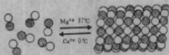
图3 微管蛋白的聚合与解聚
