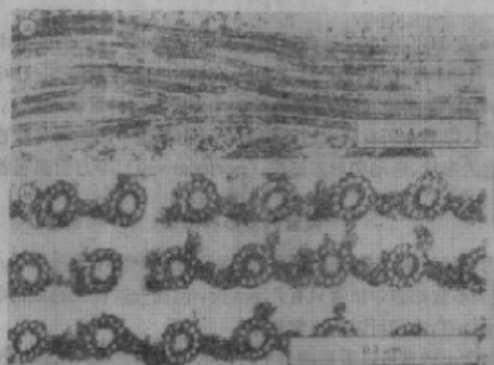
图1 电子显微镜下的微管 (a) 纵切面, (b) 横切面。
