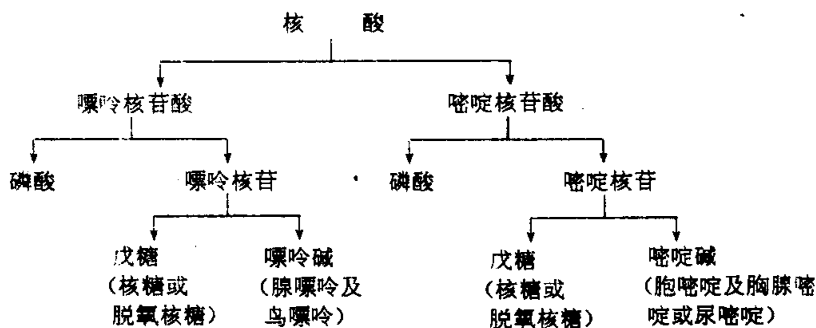
图 1-1 核酸的水解产物
