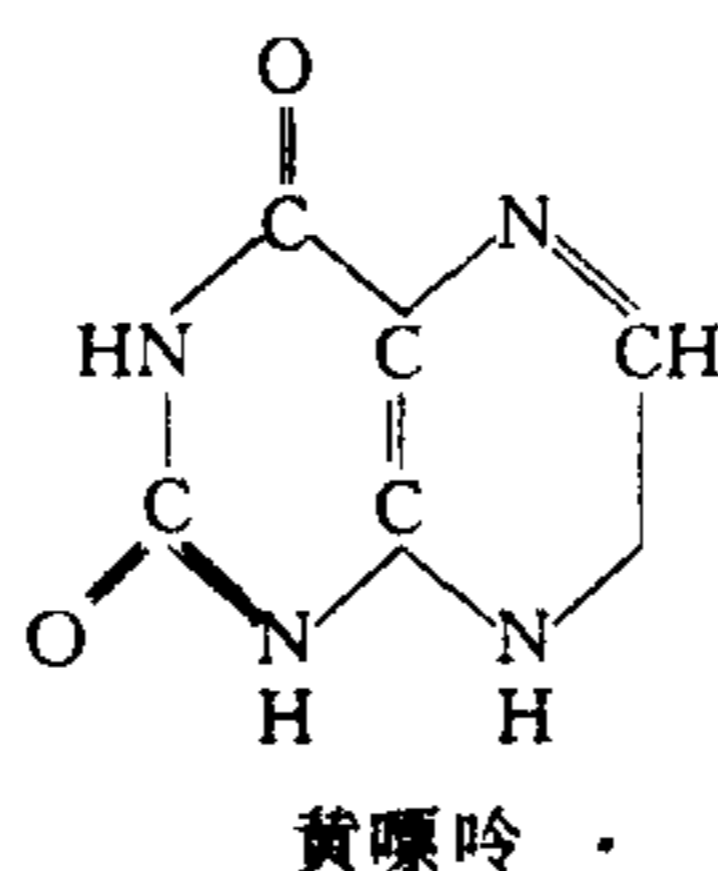
图 2-2 嘌呤碱的构造式
