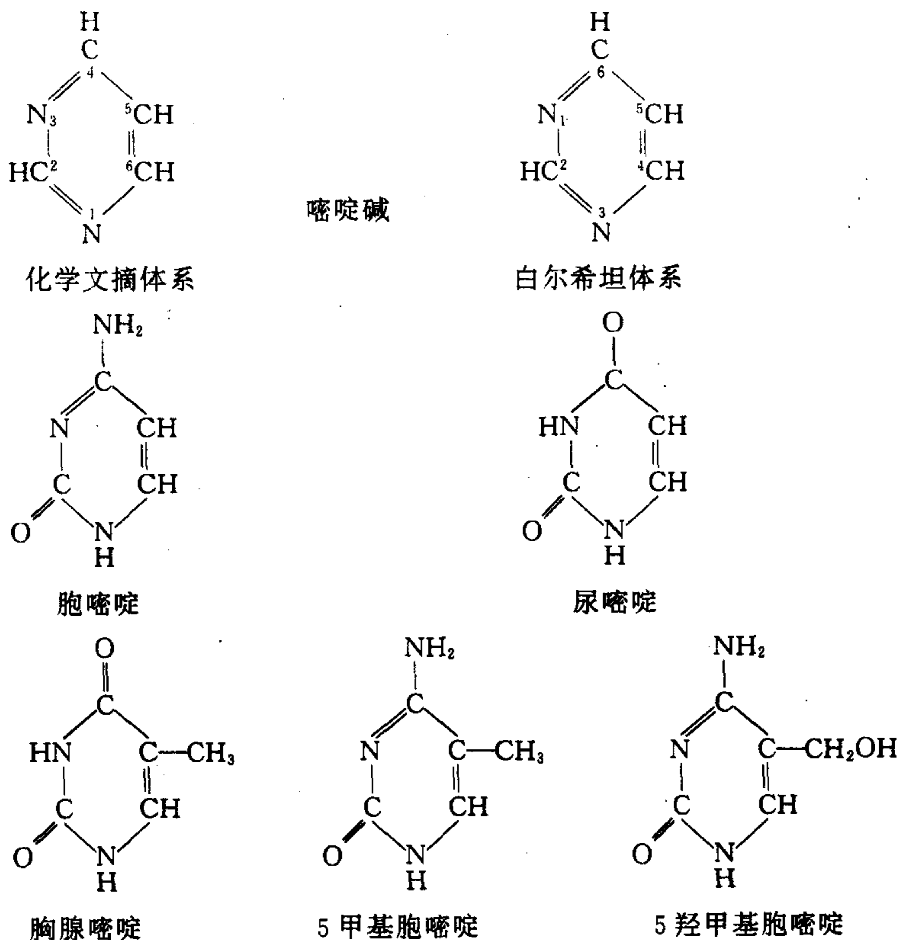
图 2-1 嘧啶碱的构造式
