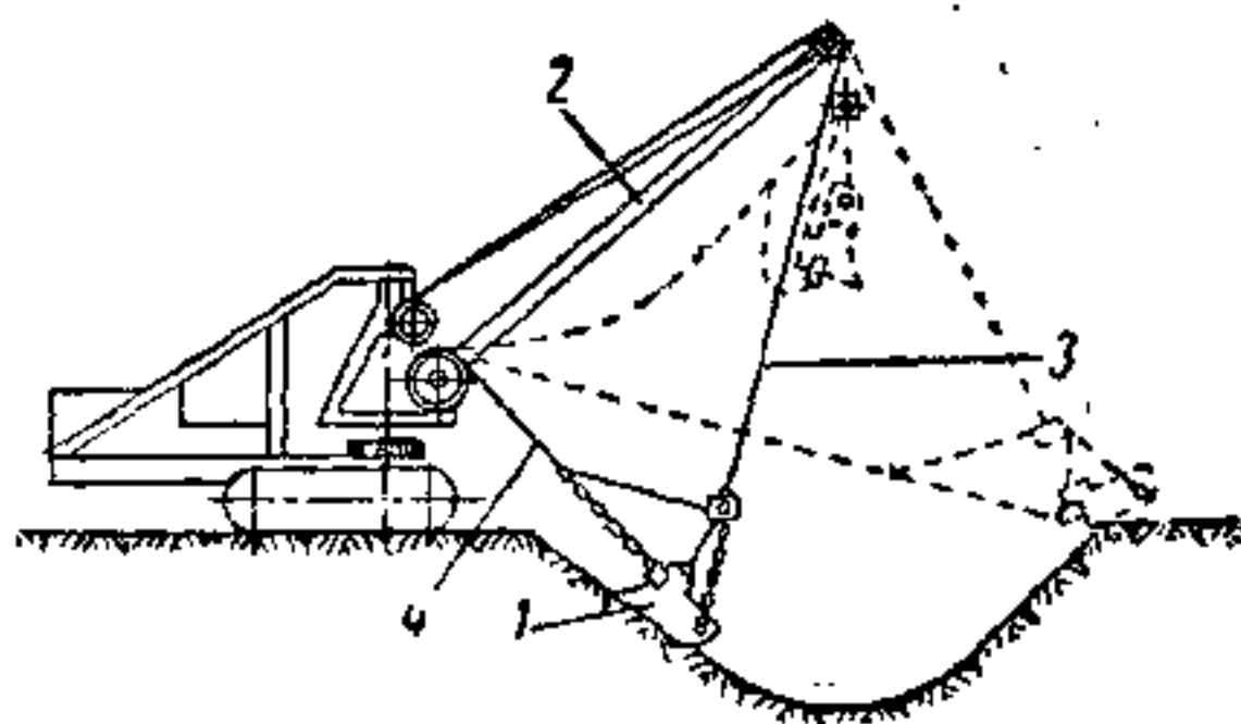
圖 3 吊斗式挖掘机
