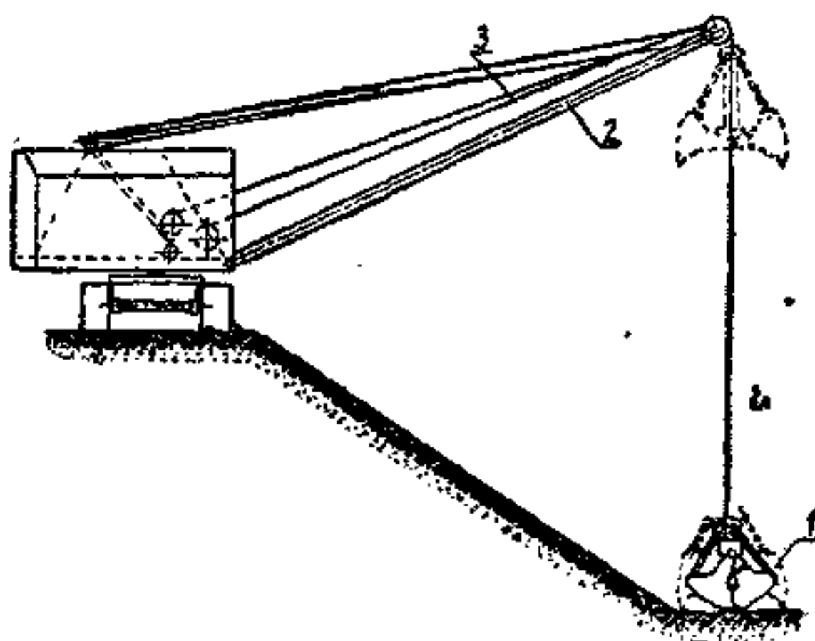
圖 4 撮斗式挖掘机
