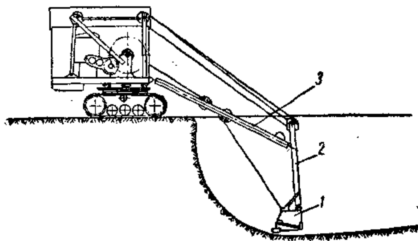
圖 2 反鏟式挖掘機
