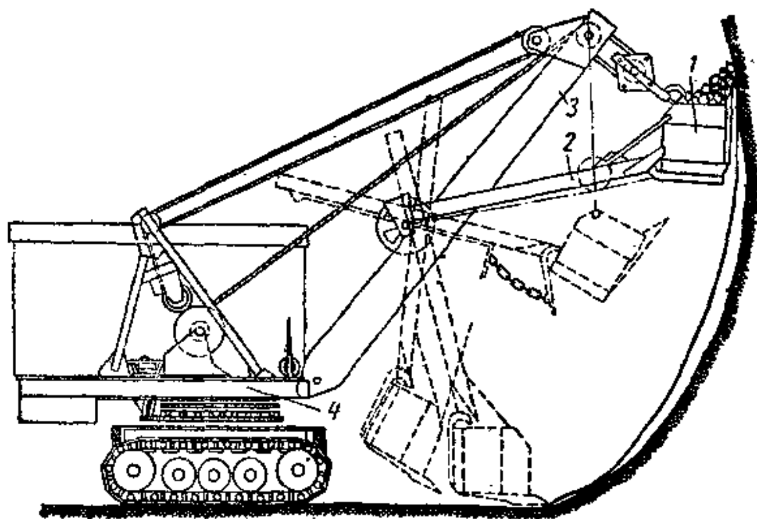
圖1 正鏟式挖掘机
