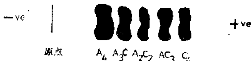
图2.3 鼠脑醛缩酶同工酶的电泳分离谱。在pH6.8的乙酸纤维素上电泳之后，电泳条浸渍于含醛缩酶底物——氮蓝四唑 (nitro blue tetrazolium) 和其它试剂的检验介质中，醛缩酶同工酶的位置以深色区带显示出来。在此反应中，醛缩酶活性导致四唑盐的有颜色的甲脎衍生物之形成 (看第八章)
