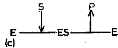
图 2.3 一底物机制的三种不同的表达图式。
