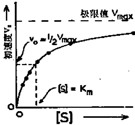
图 2.2 典型的酶促反应中,初速度与底物浓度的关系。
