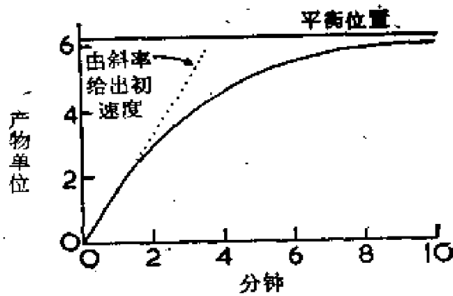
图 1.1 典型的反应-时间进程。
