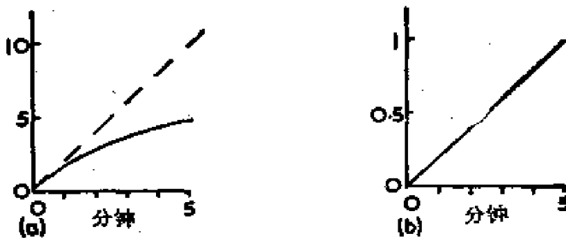
图 1.2 仪器的灵敏度和酶浓度对初速度测定的影响。
