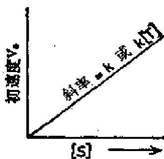
图 2.1 简单的一级或二级化学反应中，初速度与反应物浓度的关系。
