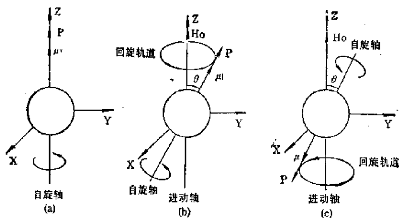
图 1-1 氢核在外磁场 H_0 中的拉摩尔进动
