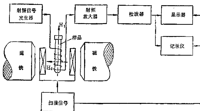
图 1-4 连续波核磁共振仪示意图
