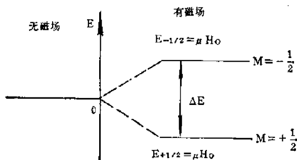
图 1-2 核磁能级分裂
