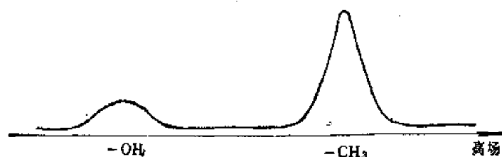
图 1-3 \text{CH}_3\text{OH} 的 NMR 波谱简图
