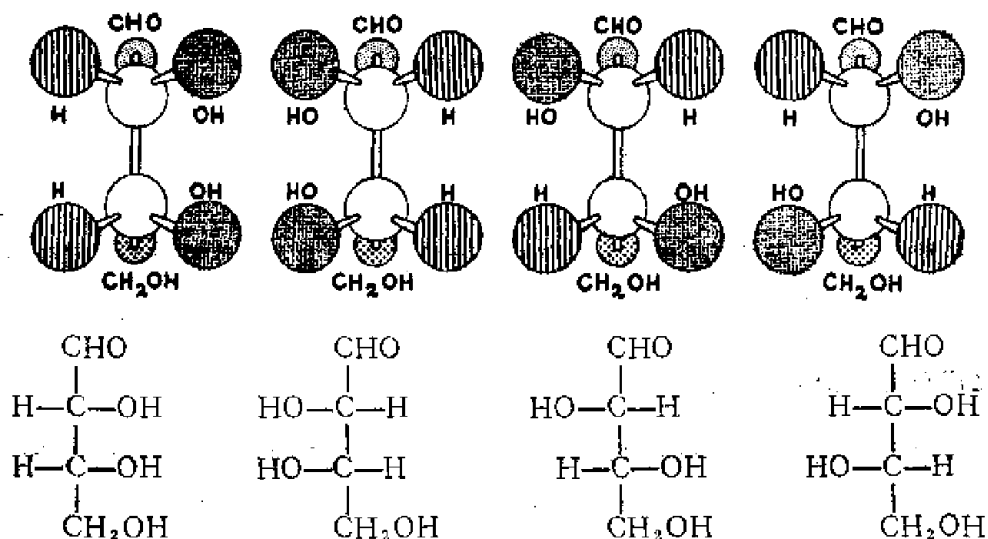
图1—2 丁醛糖：上、球和棒模型，下、Fisher投影式
