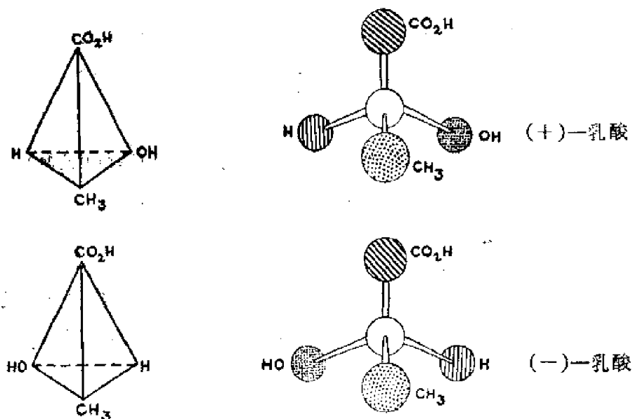
图1—1 乳酸对映体的四面体模型及球和棒模型
