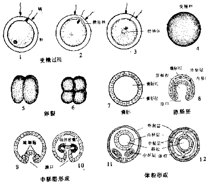
图 1—2 多细胞动物胚胎发育过程示意图 (综合 Hickman 与 Meglitsch)
