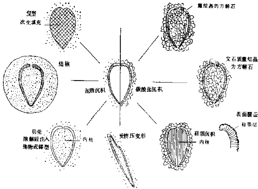
图 1—1 化石作用的可能过程 (以双壳类贝壳为例) (引自Clarkson, 1980, 稍修改)
