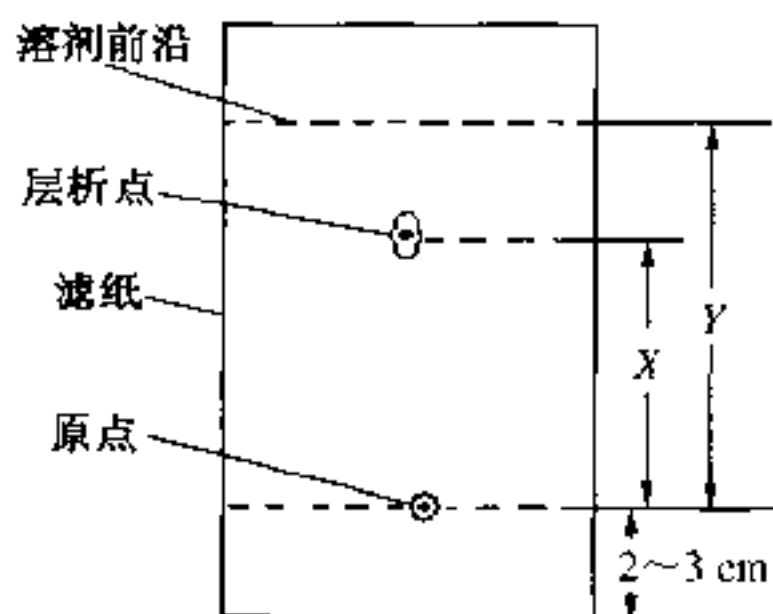
图 1-1 纸层析中的 R_f , R_f = \frac{X}{Y}
