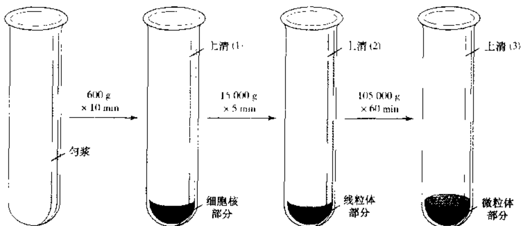
图 2-2 用差速离心分离亚细胞部分的示意图。组织(如肝脏)匀浆首先进行低速离心,得到细胞核部分(包括细胞核和没有破碎的细胞)和上清液(1)。将上清液移入(2)并进行中速离心,获得线粒体部分(包括线粒体、溶酶体和过氧化物酶体)及上清液(2)。转移上清液至(3),进行高速离心,得到微粒体部分(包括核糖体、光面粗面内质网的混合物)和最终清亮的上清液(3)。清亮的上清液相当于胞浆。对基本途径进行各种改进,一般能获得相对纯净的每一种细胞器。
