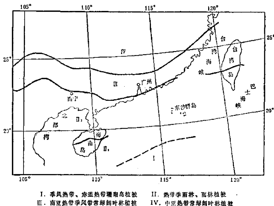
图3 南海中北部及陆缘植被图
