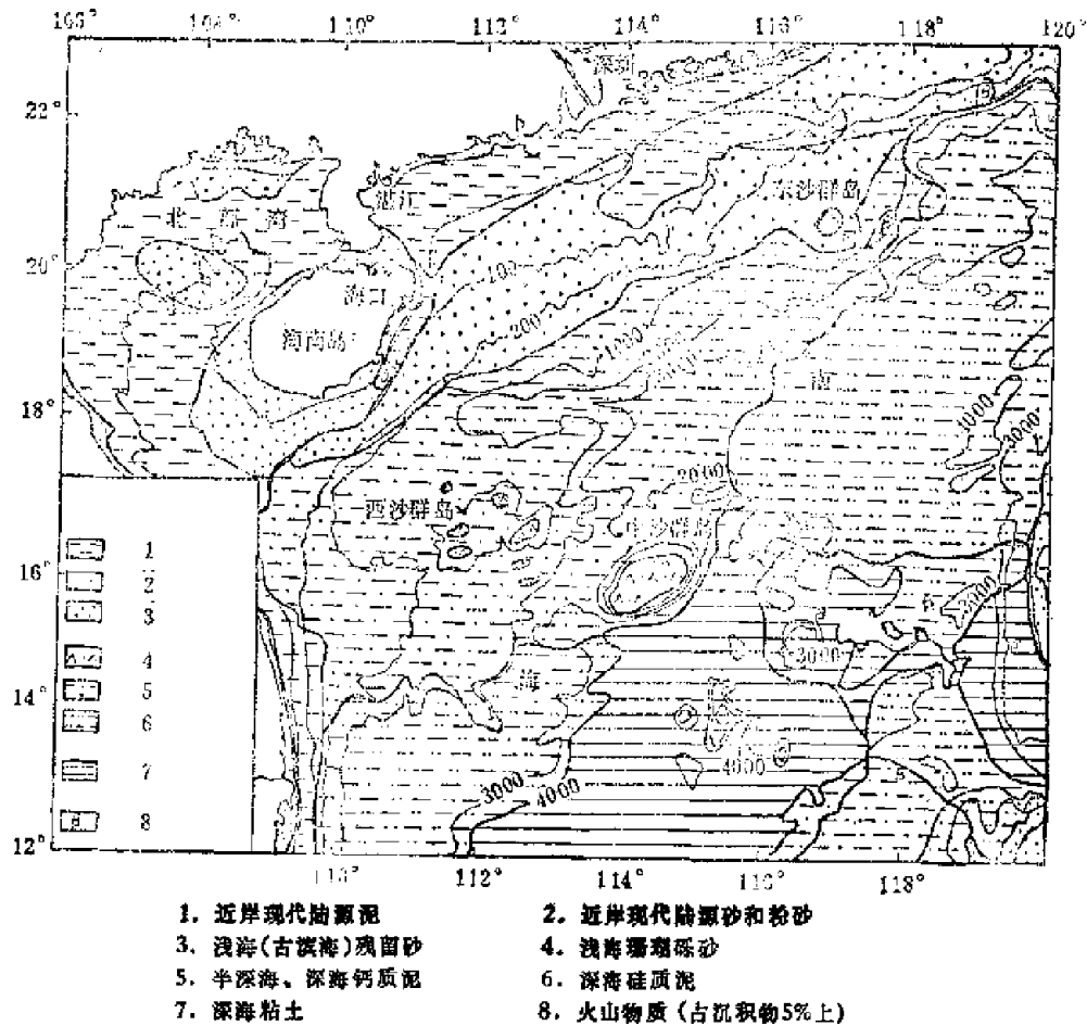
图 2 南海中北部表层沉积物类型
