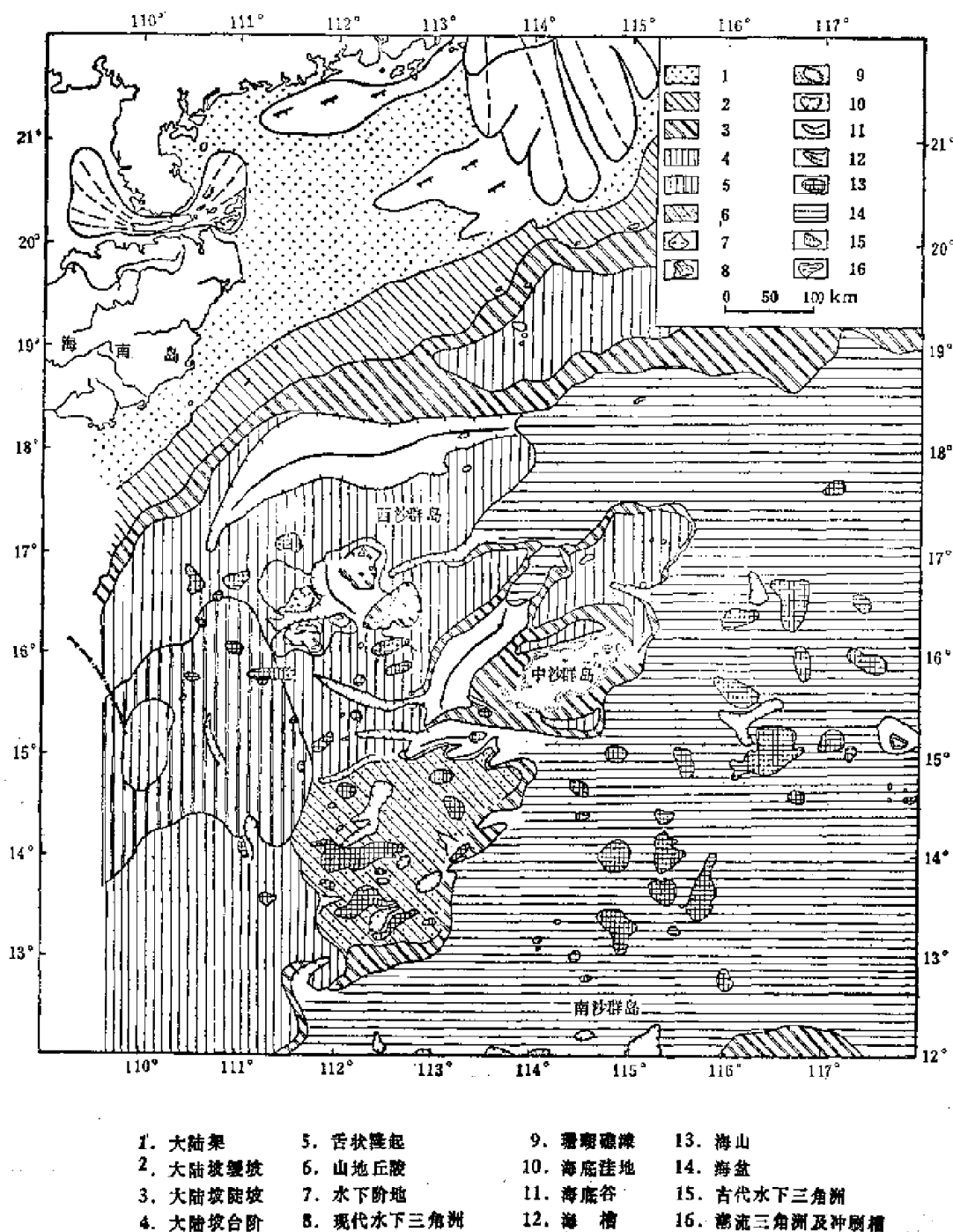
图1 南海中北部海底地貌图
