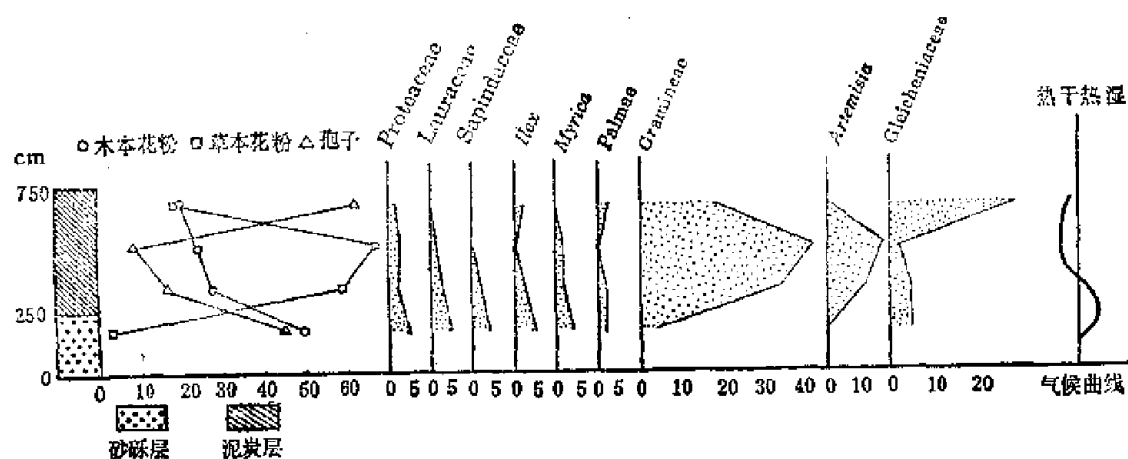
图 5 湛江组 Fe-127 剖面孢粉图式
