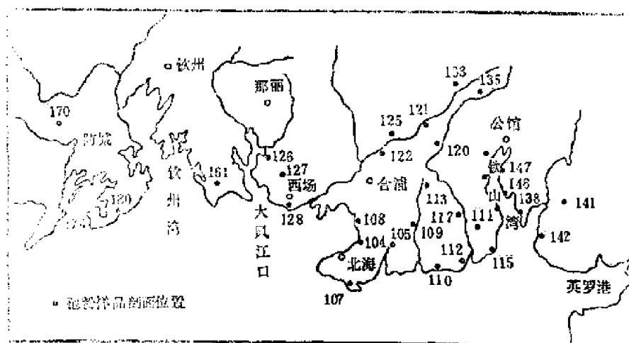
图 4 北部湾沿岸第四纪孢粉样品位置图
