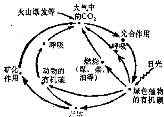
图绪-1 碳循环
