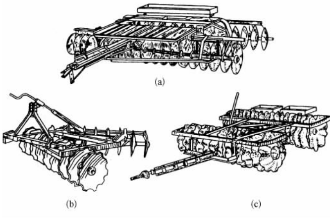
图 1-5 常用圆盘耙
