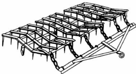
图 1-6 钉齿耙
