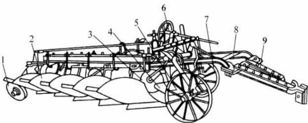
图 1-2 牵引犁
