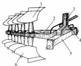
图 1-4 翻转犁
