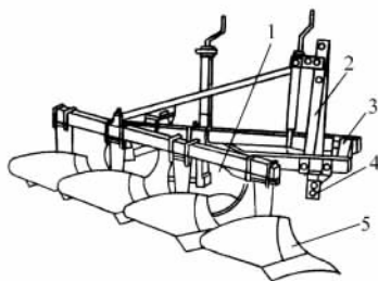
图 1-3 悬挂犁
