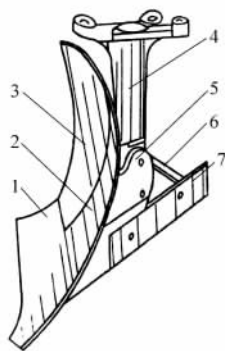
图 1-1 主犁体
