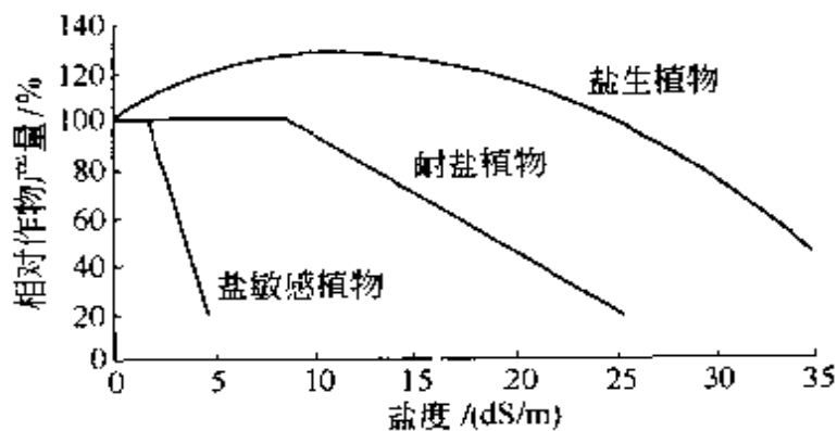
图 1-1 3 类植物对盐度的生长反应
