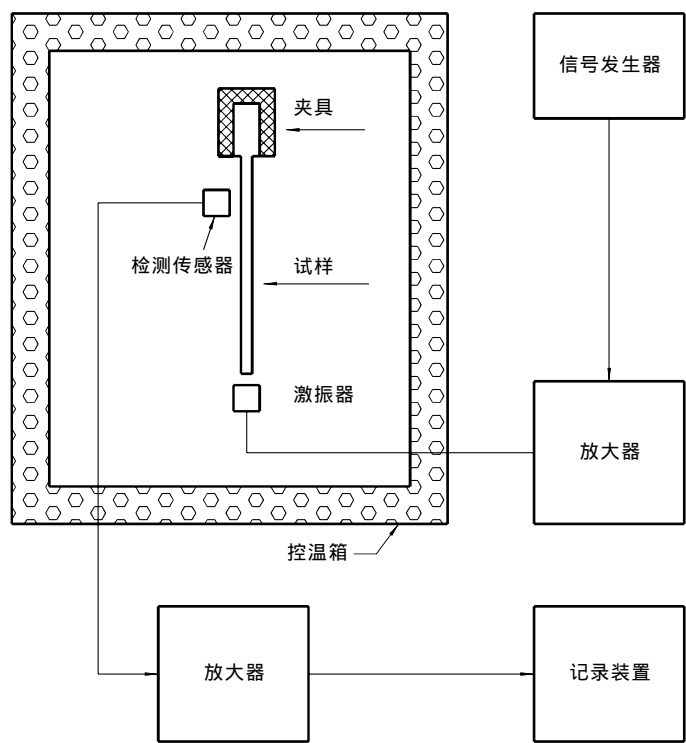
图 1 实验框图
