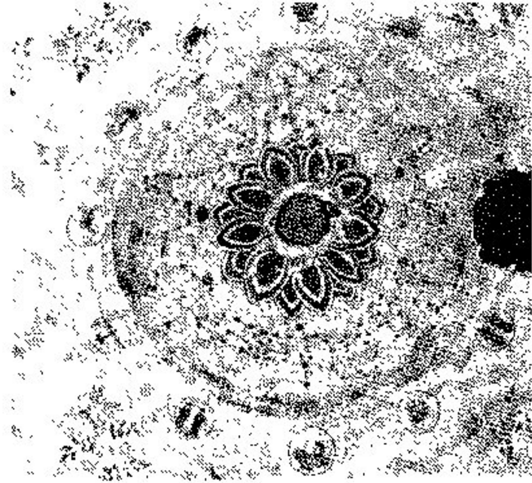
辽代星象图
