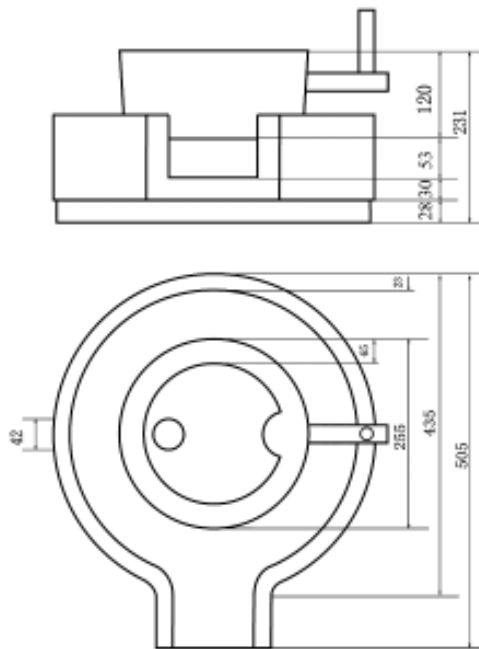
图十七 近代手牵石磨三视图
