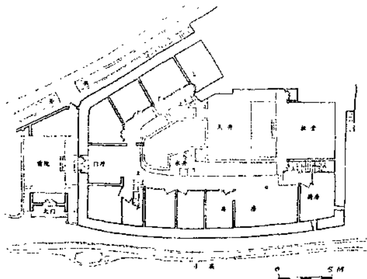
顺源楼底层平面图
