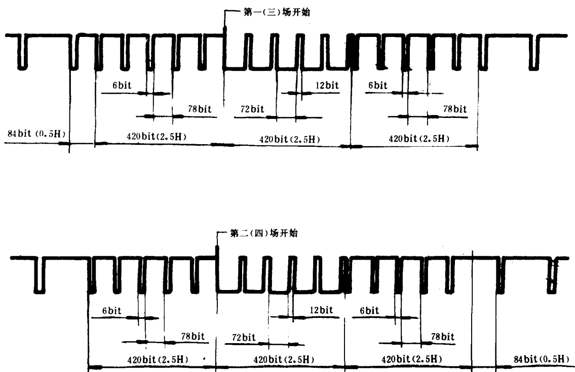
图 2 场同步信号
