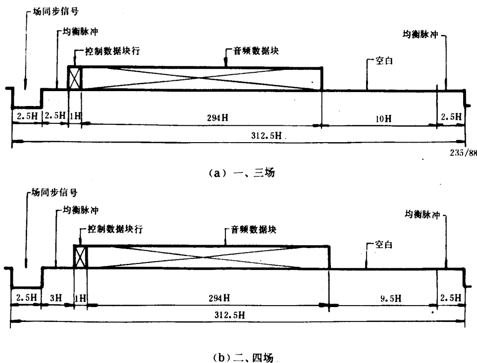
图 4 场中的配置
