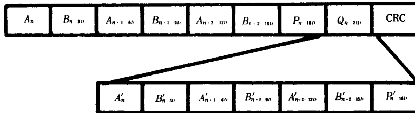
图 B1 音频数据块的组成
