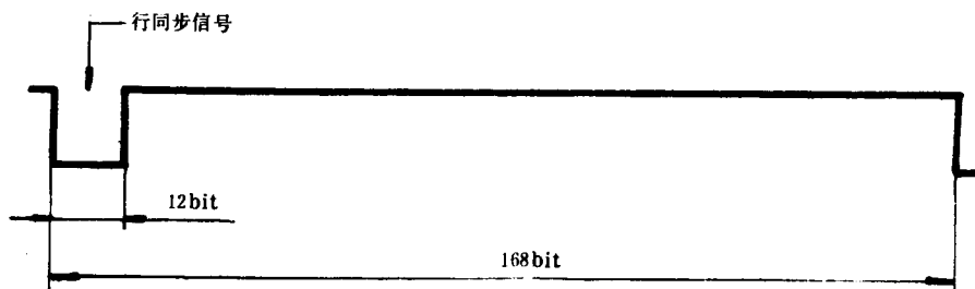
图 1 行周期
