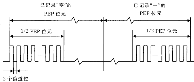
图 1 PEP 区中的相位编码调制实例
