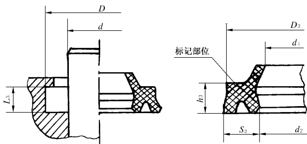
图 2 B 型密封结构型式及 B 型防尘圈
