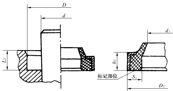
图 1 A 型密封结构型式及 A 型防尘圈
