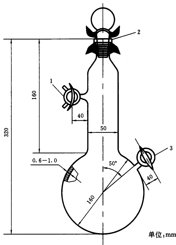
1—三向两通高真空活塞( \phi 24/32); 2—19号标准磨口; 3—直通高真空活塞( \phi 24/32)
