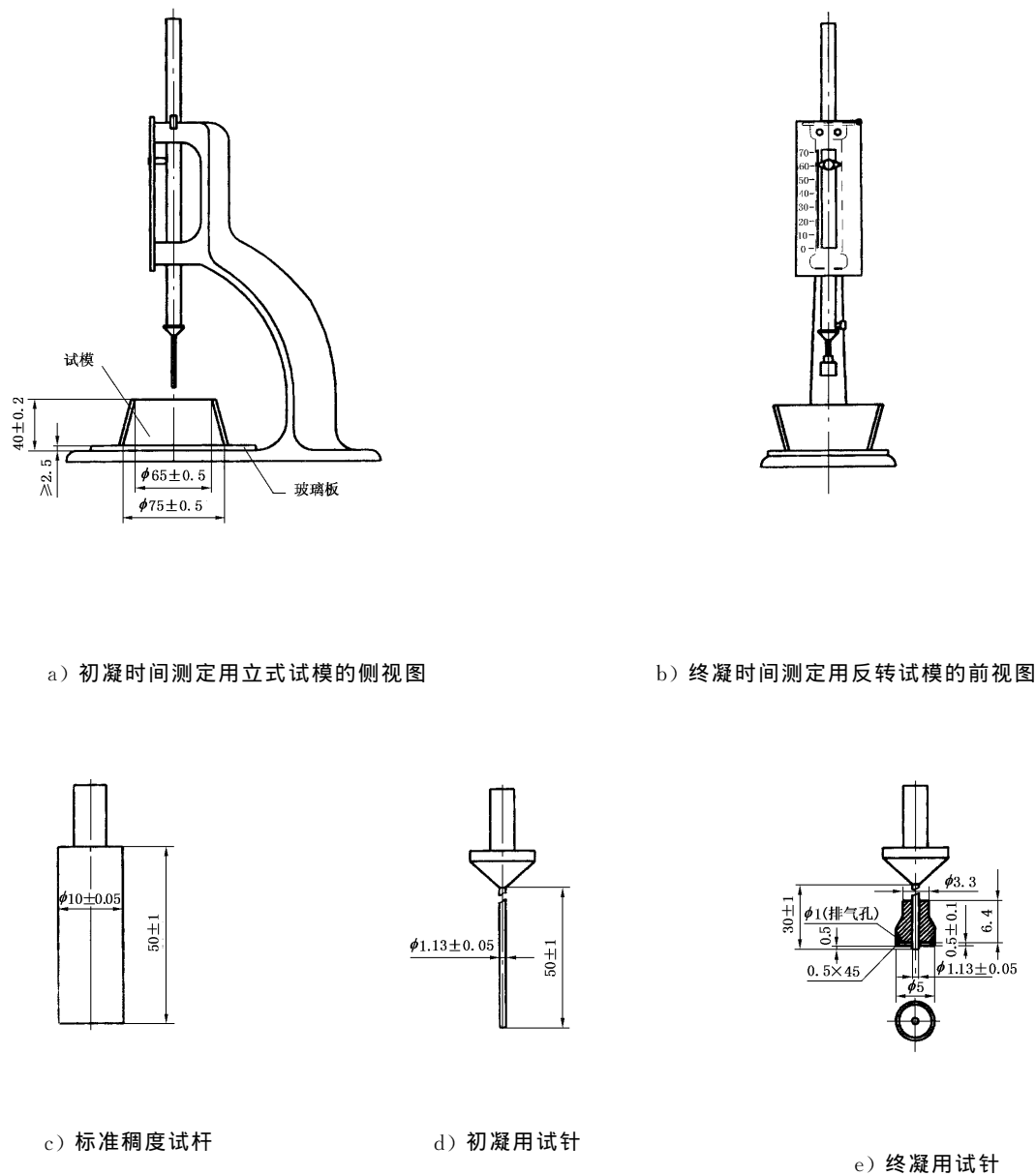
图 1 测定水泥标准稠度和凝结时间用的维卡仪
