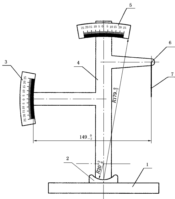
图 3 雷氏夹受力示意图
