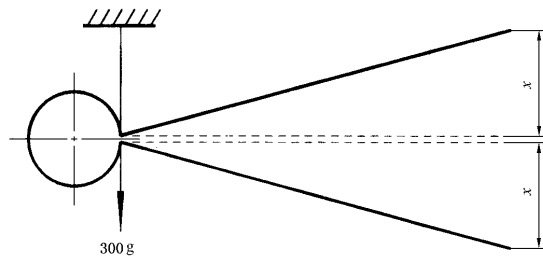
图 2 雷氏夹
