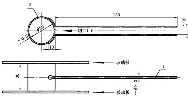
1—指针;2—环模
