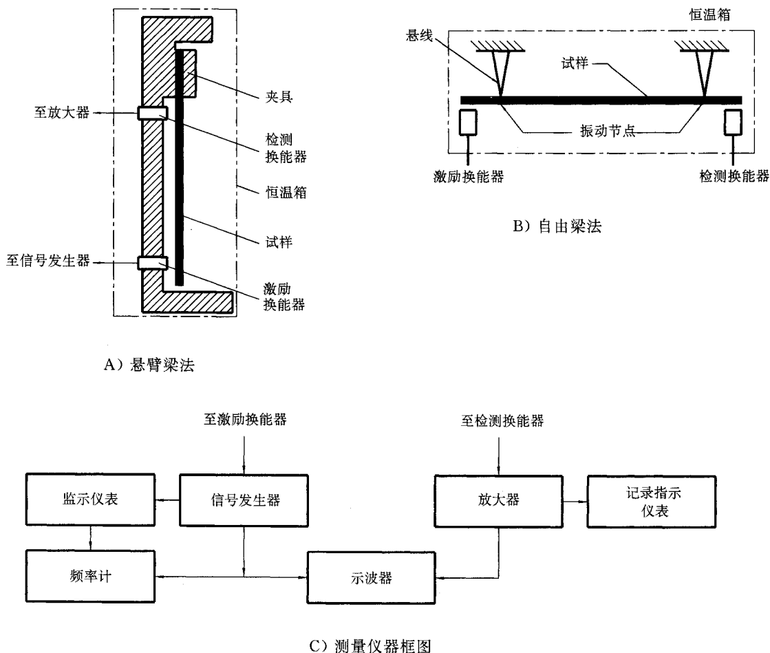
图 1 测量原理图
