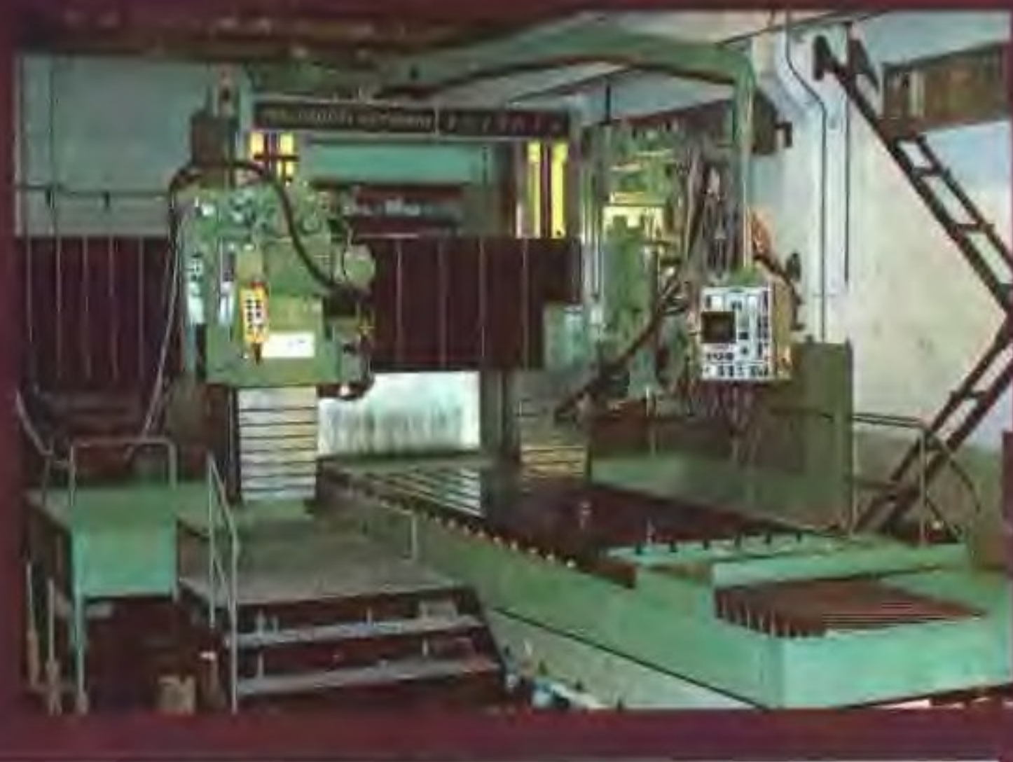
上海重型机床厂与外商合作制造的高精度工作母机 ——精密导轨磨床
