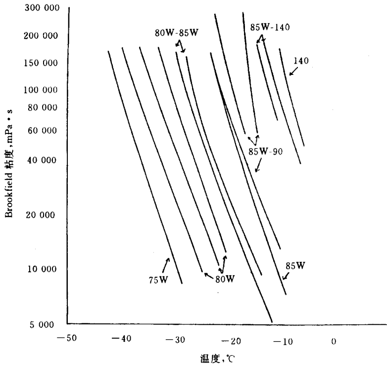
图 A1 对于典型的齿轮润滑剂 Brookfield 粘度-温度图 (指 SAE 粘度级)
