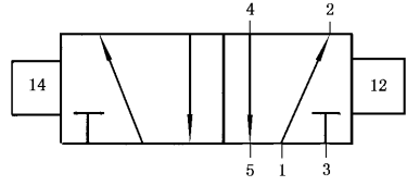
图 8 与先导控制有关的气口间的关系
