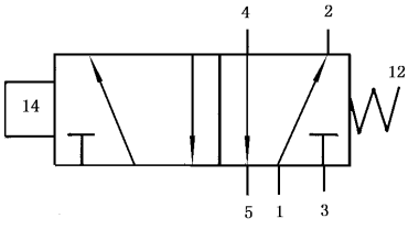
图 7 单稳态(单控)阀的强制稳态位置
