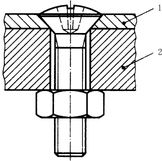
1—带沉孔的上压板；2—下压板
