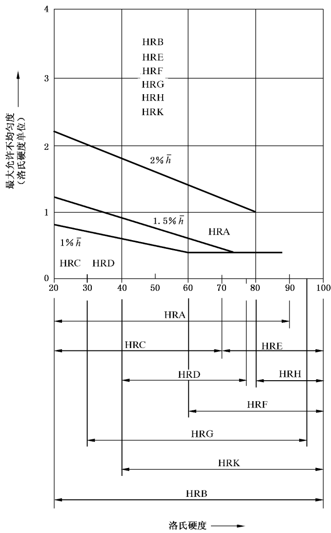
图 A.1 洛氏硬度(A、B、C、D、E、F、G、H、K 标尺)
