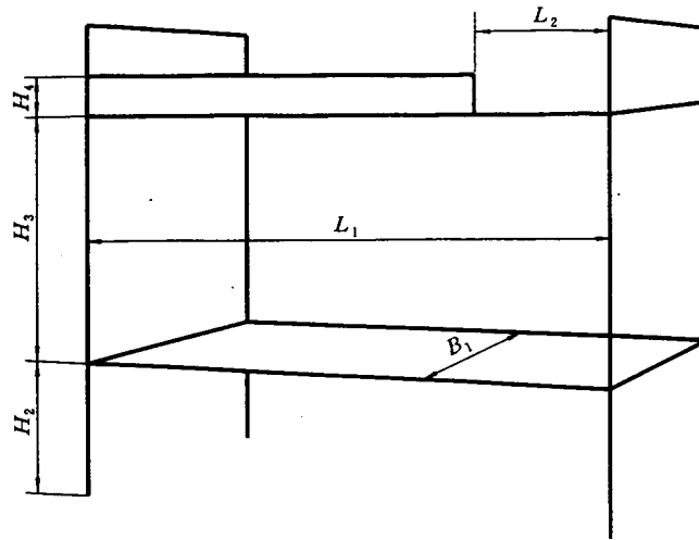
图 3 双层床主要尺寸示意图
