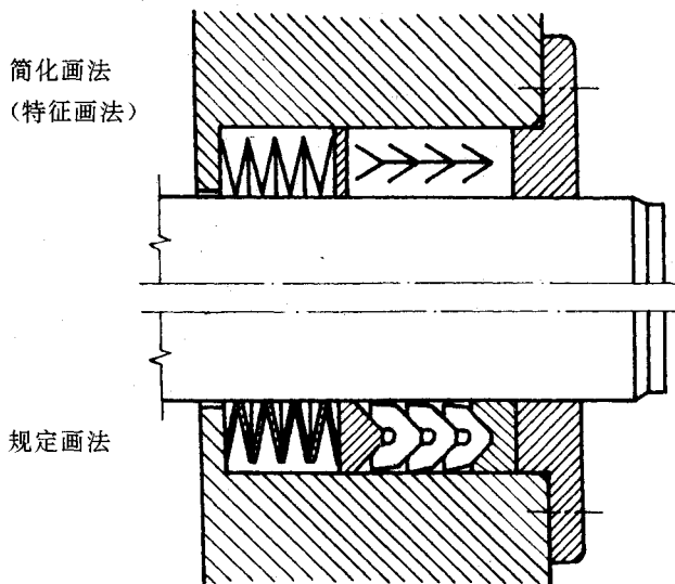
图 10 V形橡胶密封圈的应用
