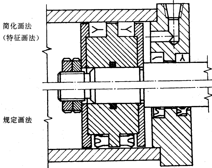
图 9 Y形橡胶密封圈、橡胶防尘圈的应用
