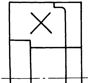
图 5 画出外形轮廓的通用画法
