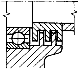
图 12 迷宫式密封的应用
