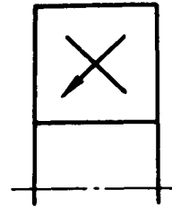
图 4 指出密封方向的通用画法
