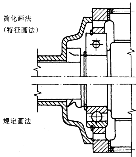
图 11 橡胶防尘圈的应用
