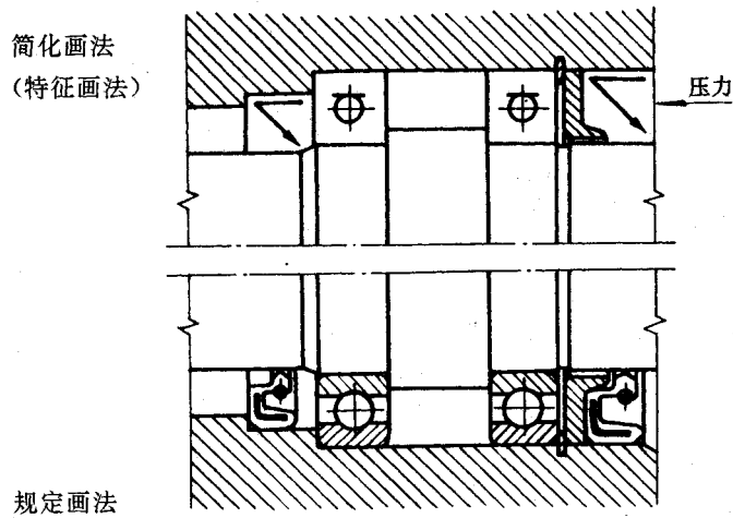
图 7 旋转轴唇形密封圈的应用
