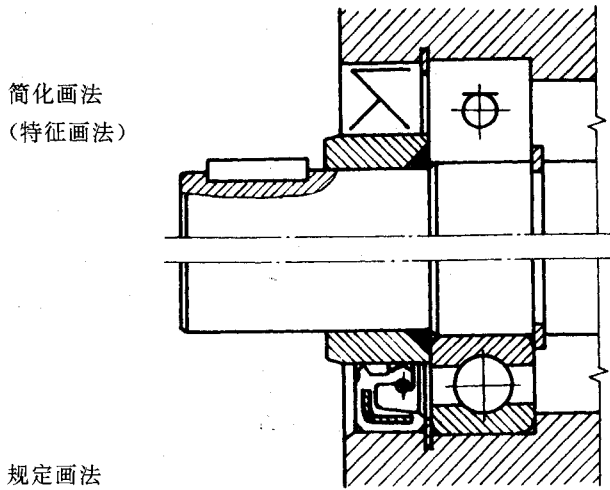
图 8 带副唇的旋转轴唇形密封圈的应用
