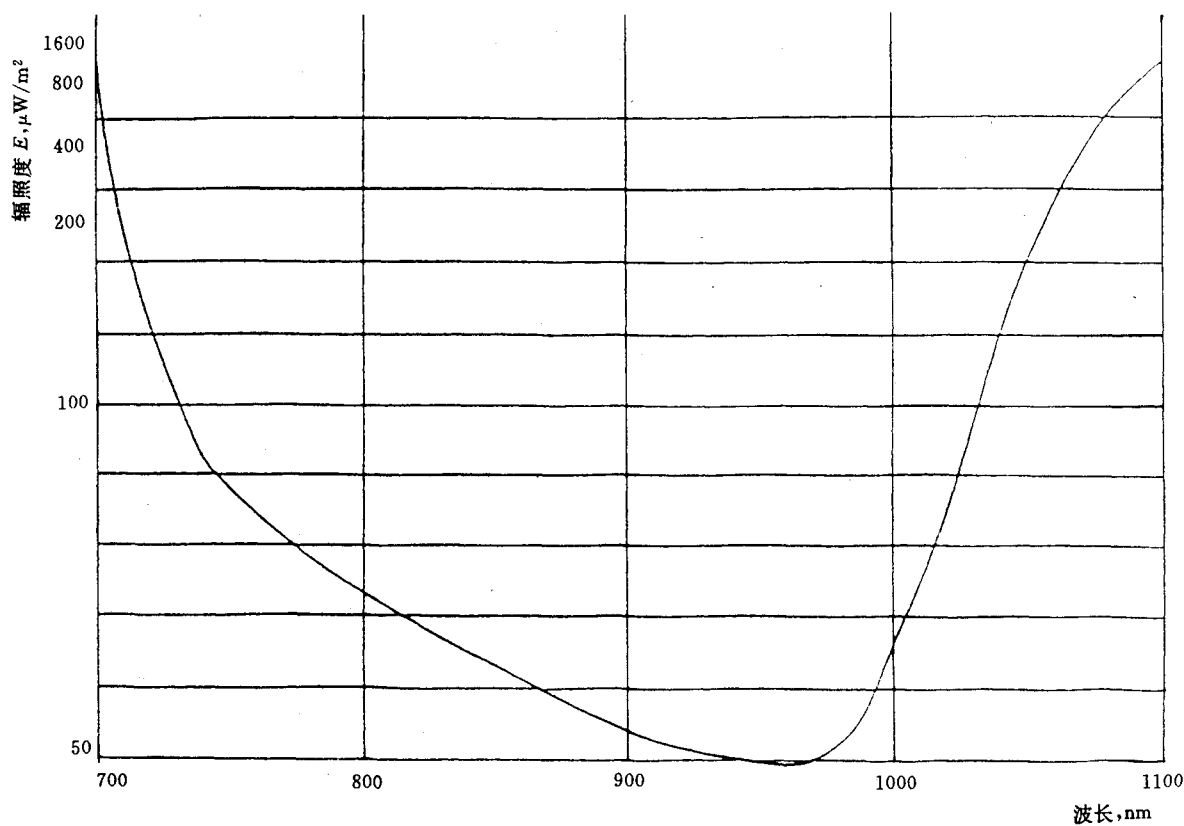
图 5 最大允许干扰辐射照度/波长关系曲线
