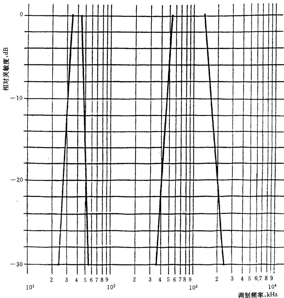
图 4 典型红外遥控接收器响应特性
