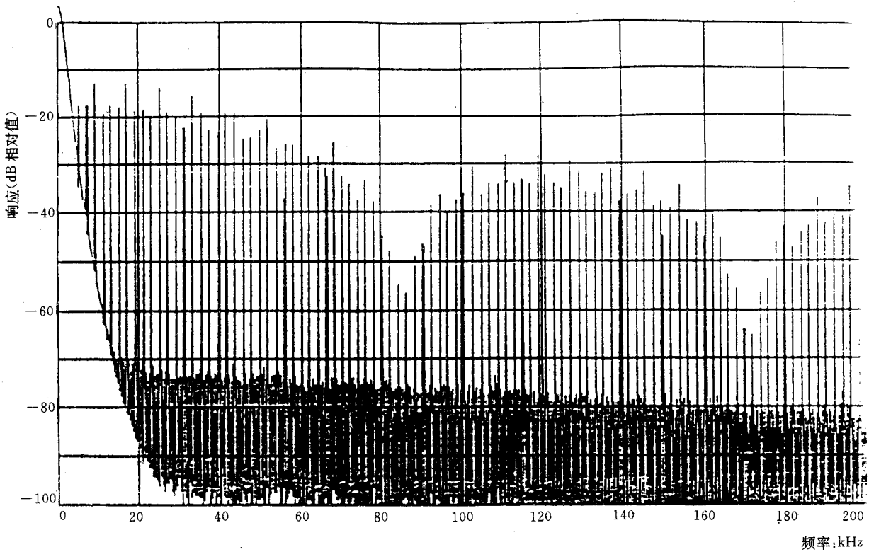
(a) 频谱
