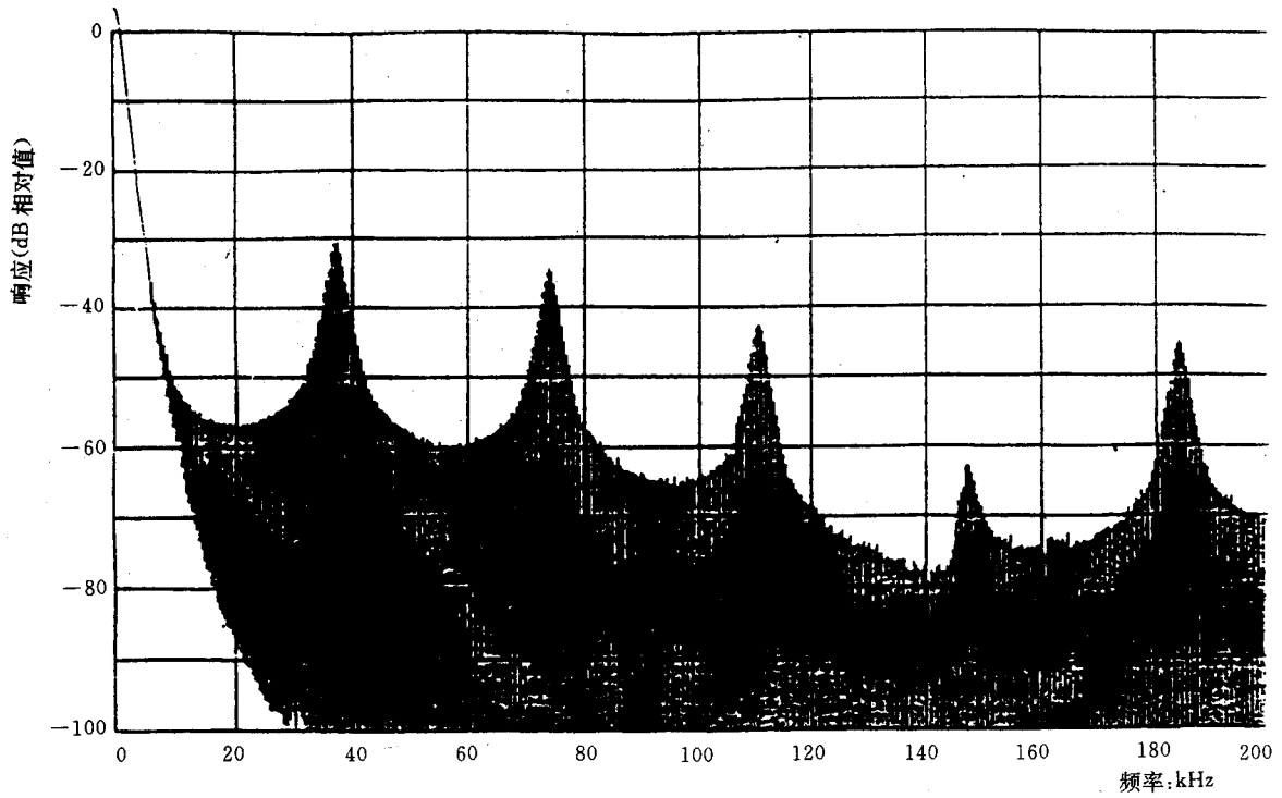
(a) 频谱
