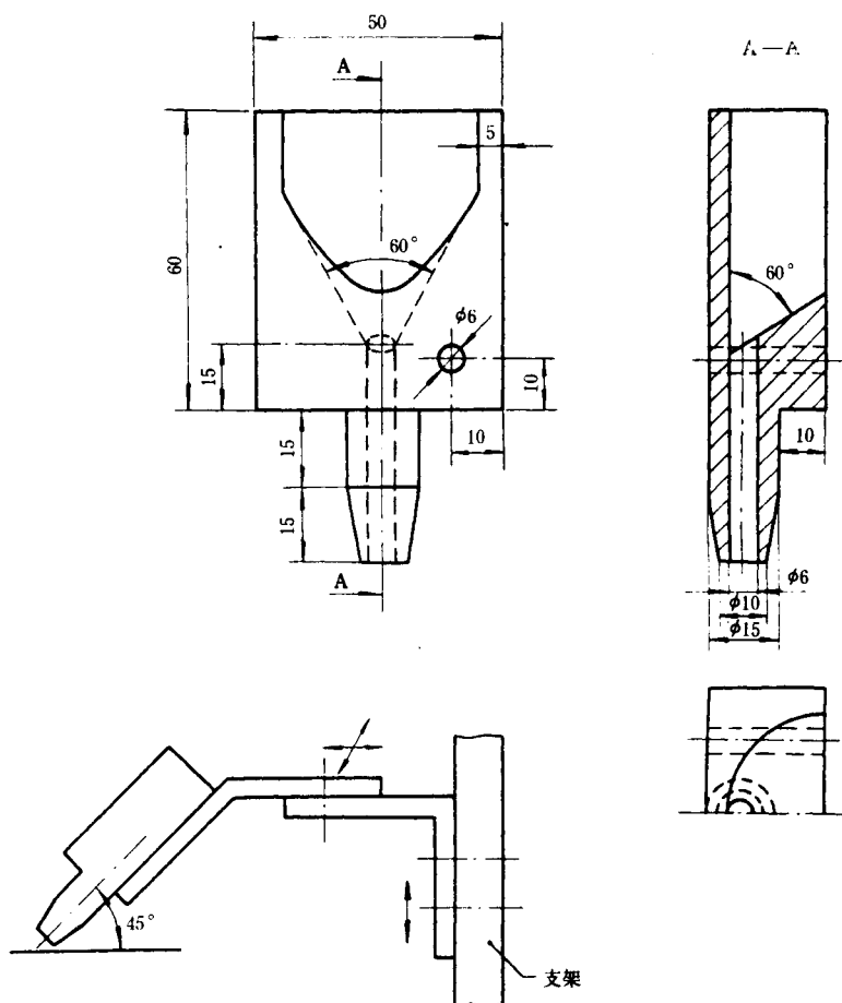
图 A3 熔滴导向机构
