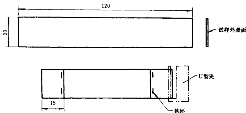
图 A6 试样
