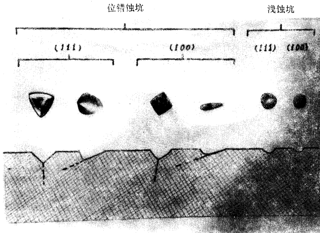
图 2 典型的位错蚀坑和浅蚀坑
