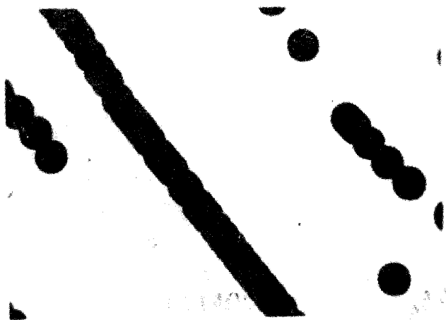
(b) (100)晶面上的小角度晶界 续图 4
