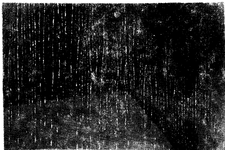
图 8 层错
