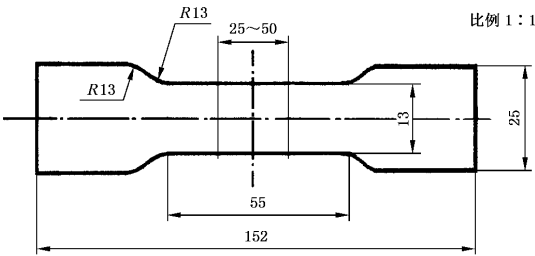
图 1 裁刀尺寸示意图
