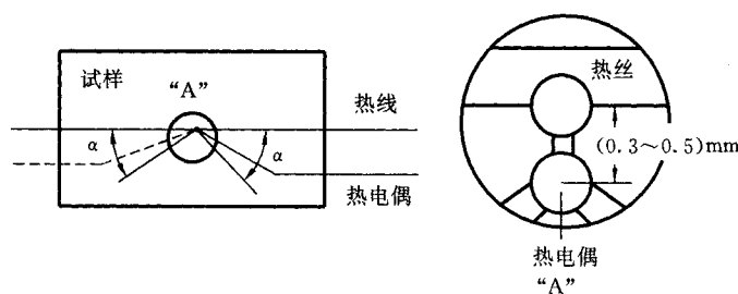
图 3 测量探头及其布置示意图
