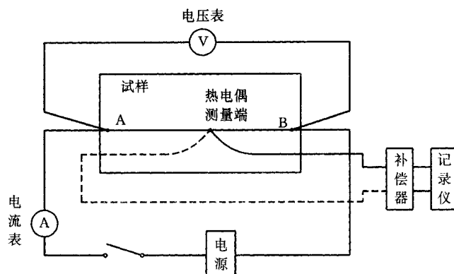
图 1 带补偿器的测定电路示意图
