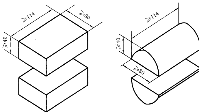
图4 试样尺寸示意图
