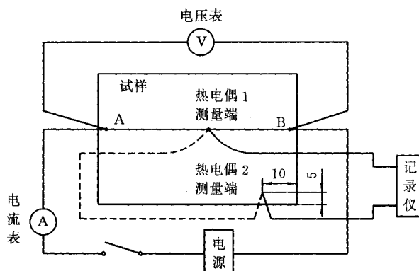
图 1 带补偿器的测定电路示意图
