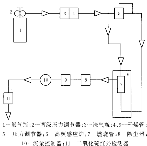
图 1 红外线吸收定硫仪装置图
