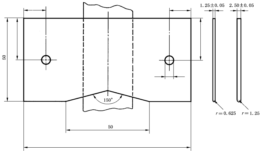
详图 A
