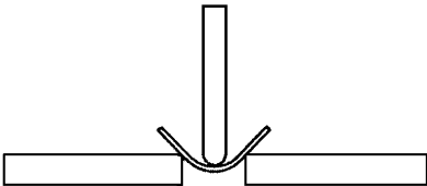
图 2 边缘撕裂夹具
