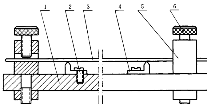
1—底座;2—螺钉;3—试样;4—电位端子; 5—电流端子;6—压紧螺钉
