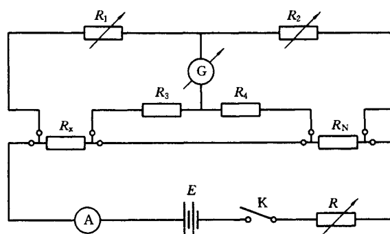
G—检流计;A—安培表; R_1 、 R_2 —电桥比较臂电阻; R_3 、 R_4 —电桥比率臂电阻; R —可变电阻; R_x —试样 电阻; R_N —标准电阻; E —稳流电源;K—闸刀开关
