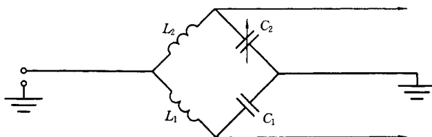
图 5 交流电桥电路图
