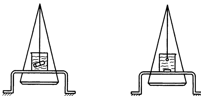
图 1 水中称量示意图
