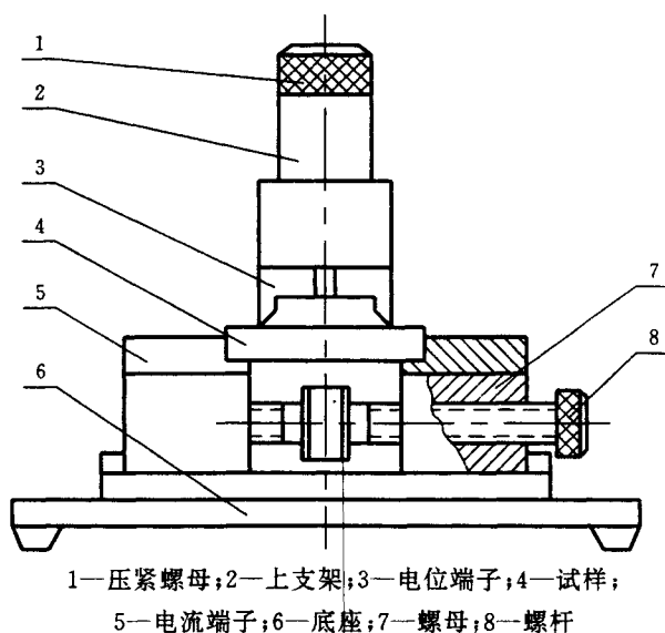
图 3 50 \text{ mm} \times 10 \text{ mm} \times h \text{ mm} 试样夹具示意图
