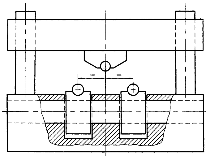
图 6 抗弯夹具示意图
