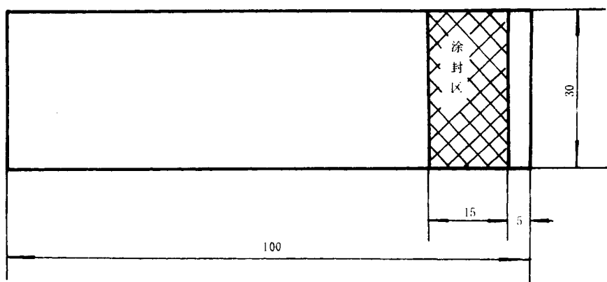
图 1 试样及涂封
