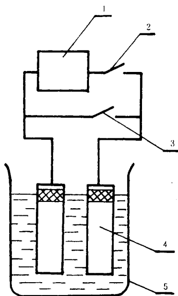
图 2 偶对配置及电连接
