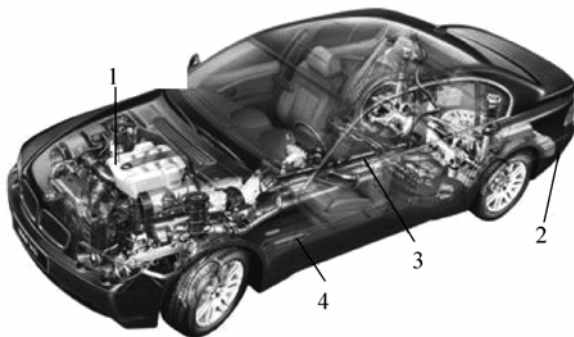
图 1-3 轿车的总体结构
