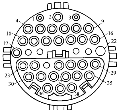
图 2-3 38 孔诊断座
