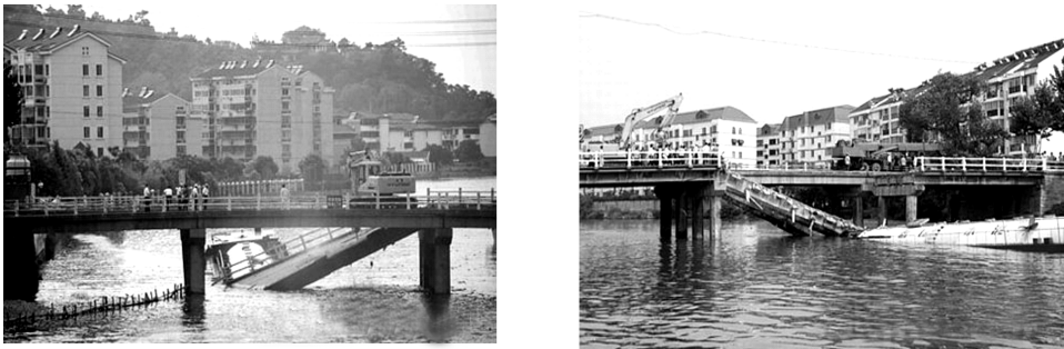
图 1-3 江苏昆山大洋桥倒塌现场照片(来自互联网)
