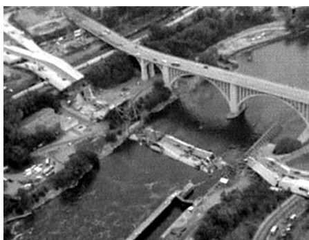
图 1-5 明尼阿波利斯大桥倒塌现场照片(来自互联网)
