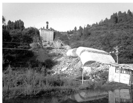
图 1-4 凤皇县堤溪大桥倒塌现场照片(来自互联网)
